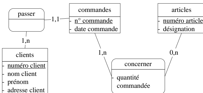
FIG. 21 – Schéma entités-associations normalisé obtenu à partir du graphe de couverture minimale
